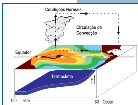
Figura 2.33. Circulação observada no Oceano Pacífico Equatorial em anos sem a presença do El Niño ou La Niña , ou seja, anos normais. A célula de circulação com movimentos ascendentes no Pacífico Central/Ocidental e movimentos descendentes no oeste da América do Sul e com ventos de leste para oeste próximos à superfície (ventos alísios, setas brancas) e de oeste para leste em altos níveis da troposfera é a chamada célula de Walker. No Oceano Pacífico, pode-se ver a região com águas mais quentes representadas pelas cores avermelhadas, e as mais frias pelas cores azuladas. Pode-se ver também a inclinação da termoclina, mais rasa junto à costa oeste da América do Sul e mais profunda no Pacífico Ocidental.
