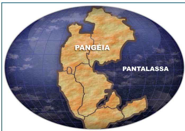
Figura 2.16. Pangéia e Pantalassa: configuração dos continentes e oceanos há cerca de 200 milhões de anos.
